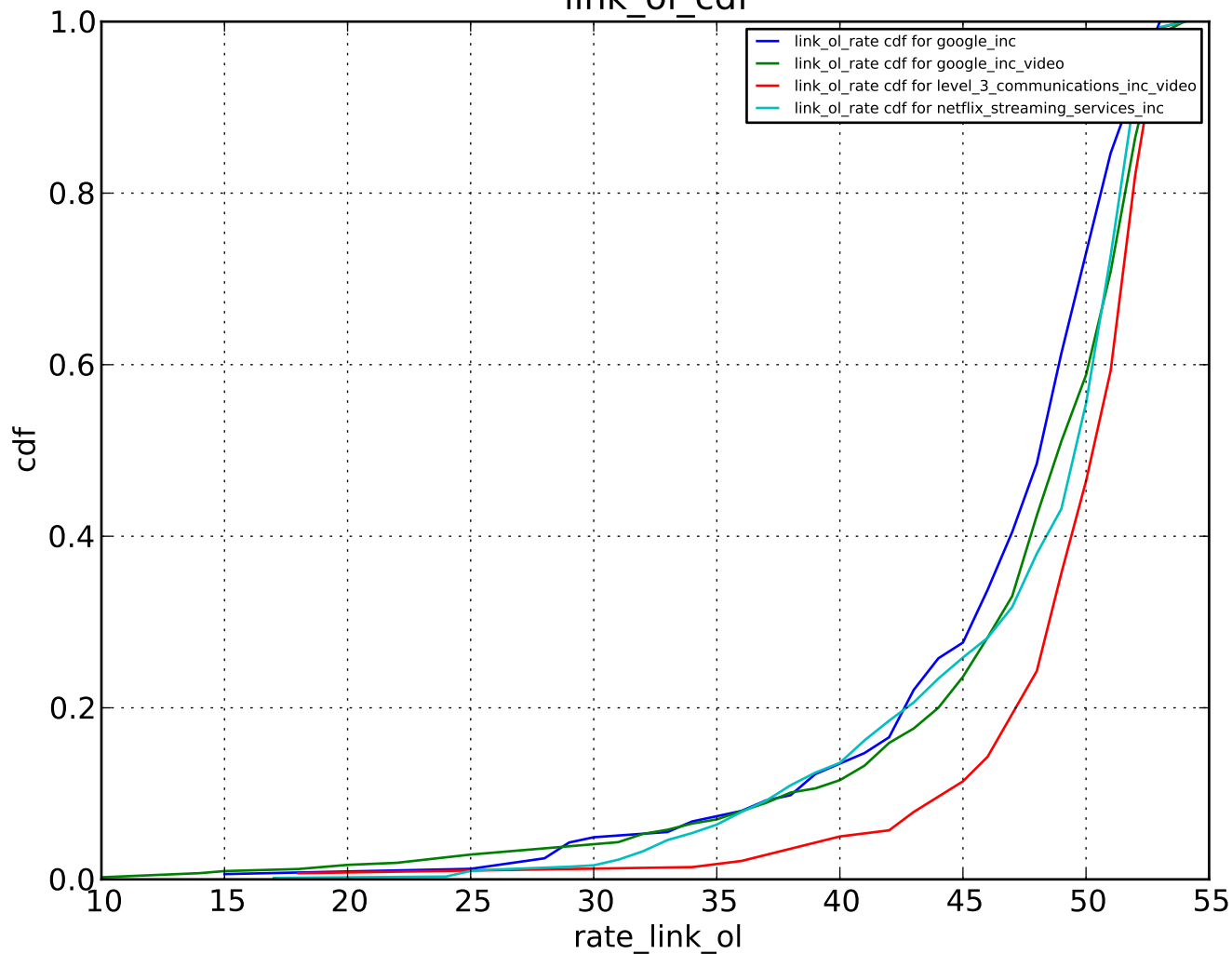
link_ol_cdf
