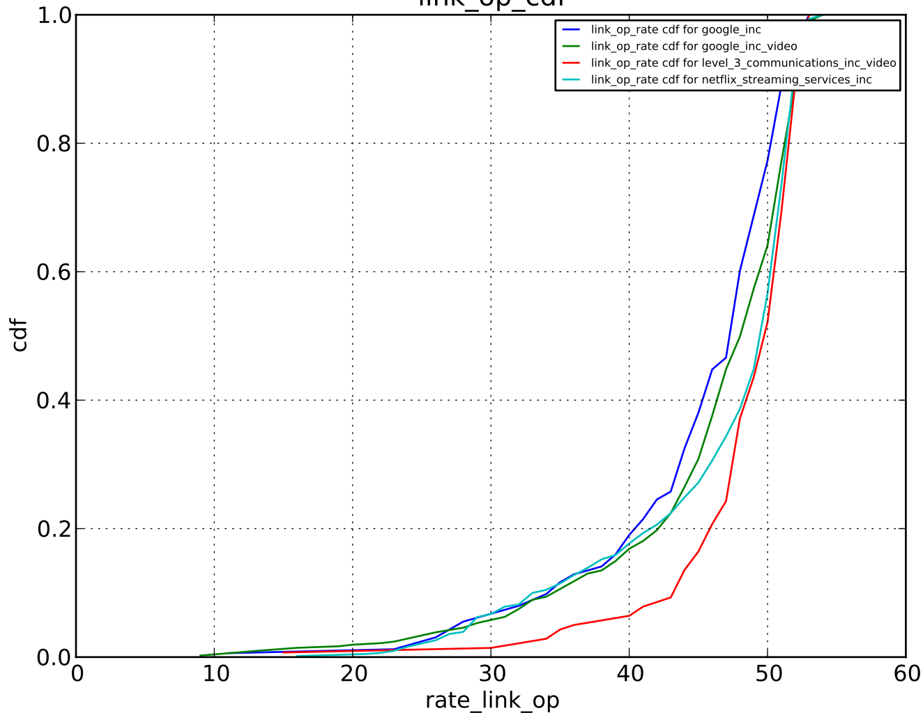
link_op_cdf
