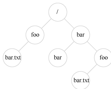
图 39.1 目录树示例
